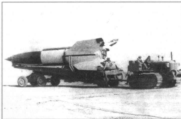
Транспортировка грунтового лафета-установщика 1Н / 8У22 ракеты Р-1 к одному из первых пусков, полигон Капустин Яр
