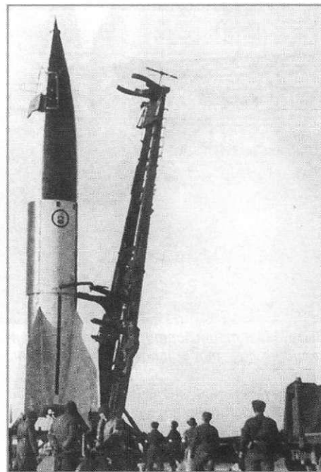
Подготовка ракеты Р-1 к одному из первых пусков, полигон Капустин Яр
