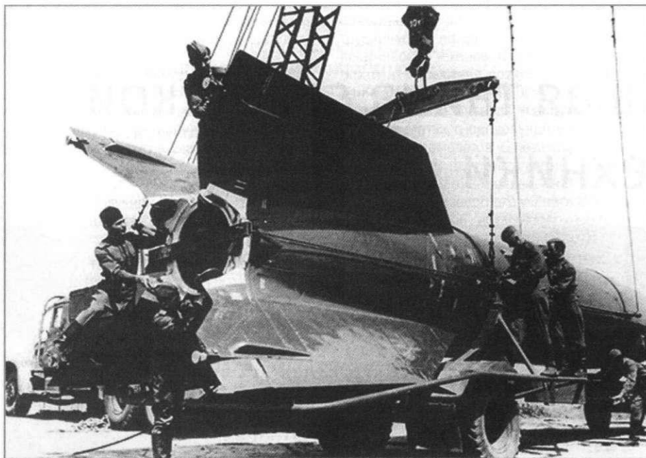
Ракета P-1 на транспортере-подъемнике
