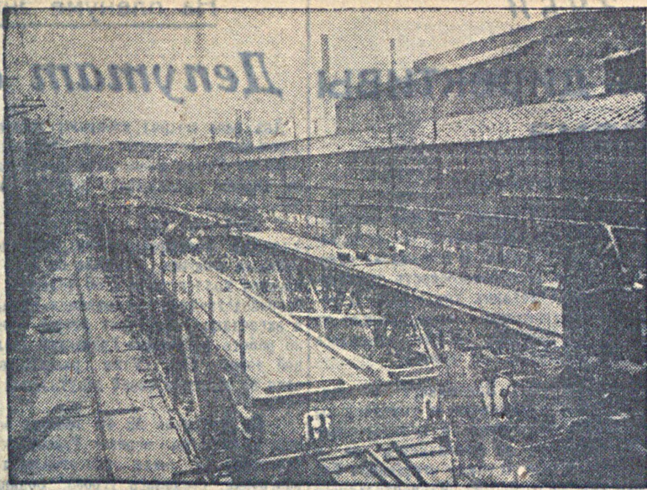
Краматорский завод тяжелого машиностроения им. Орджоникидзе (Донбасс) производит сборку мостов для строительства канала Волга—Москва. На снимке: бригада тов. Бороменского, прекриванного Наркомтажпромом Мотоциклом, за сборкой ферм моста. Совфото.
