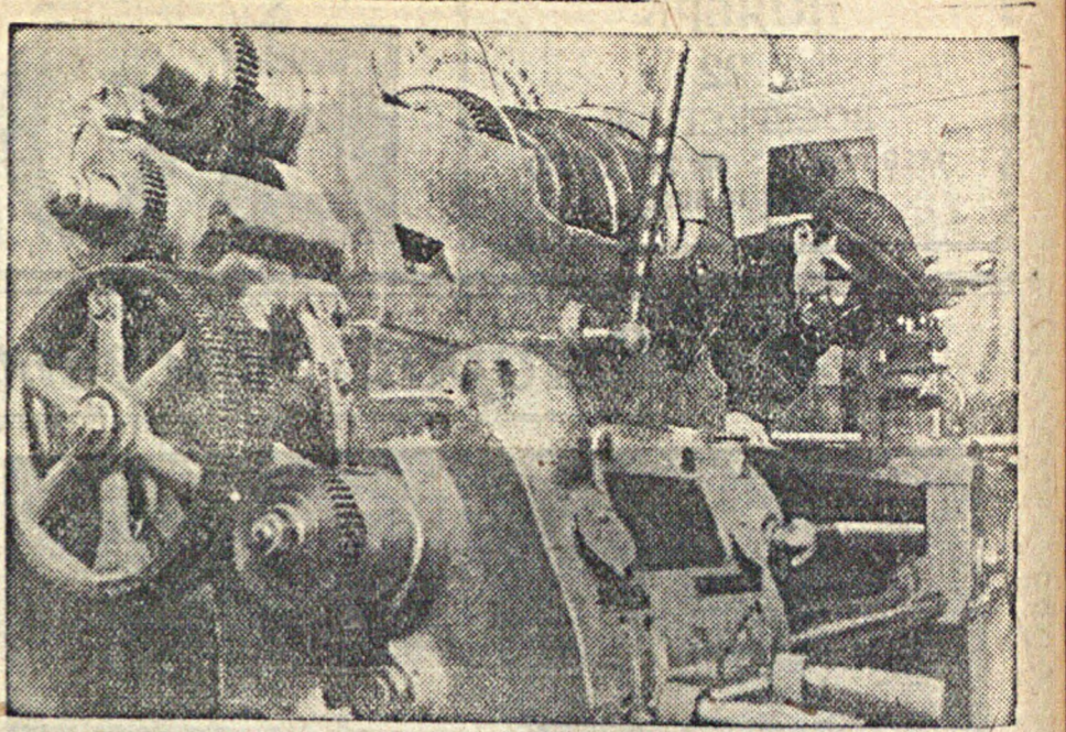
С республиканской промышленной выставки. На снимке: токарно-винторезный станок ТВ-2 производства Гримского завода «Рекорд».
