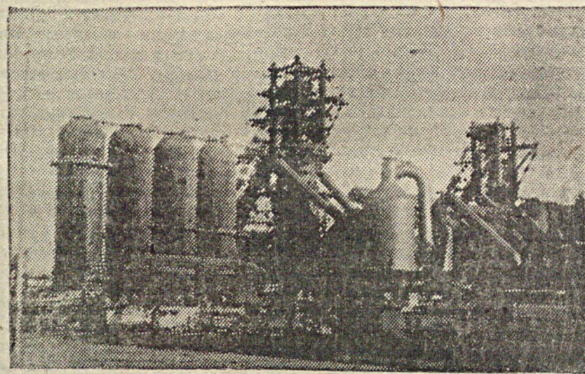
На Новотульском металлургическом заводе заканчивается строительство дома № 2 с полезным объемом печи в 930 кубических метров. На снимке: строящийся дома № 2 (слева).
