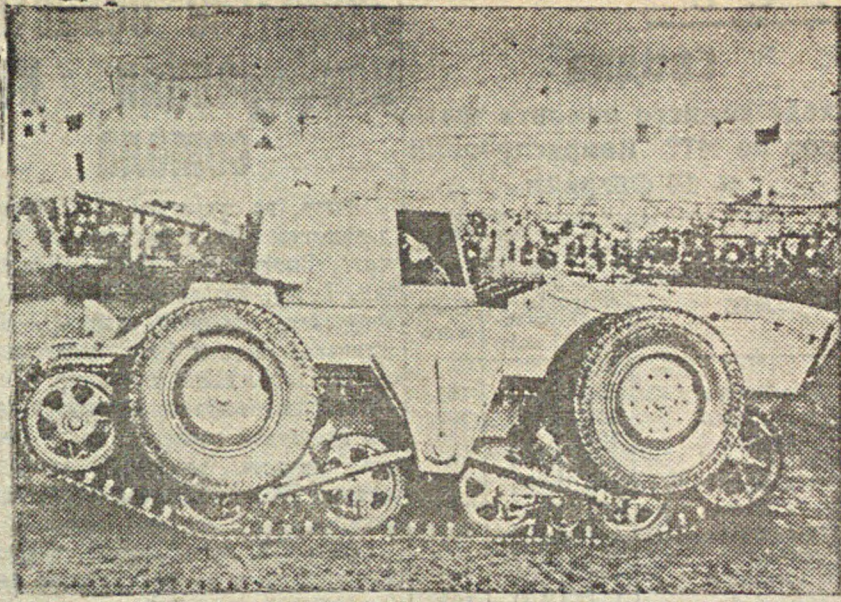
В шведской армии введены комбинированные танки новейшей конструкции. Поворотом рычага внутри танка можно в 18 секунд перевести машину с гусеничного хода на колеса. На гусеницах танк достигает скорости 38-40 км. в час, на колесах — 75 км. в час. Танк вооружен пулеметом и 3-мя скорострельными пушками, обслуживаемыми командой в 3 человека.
